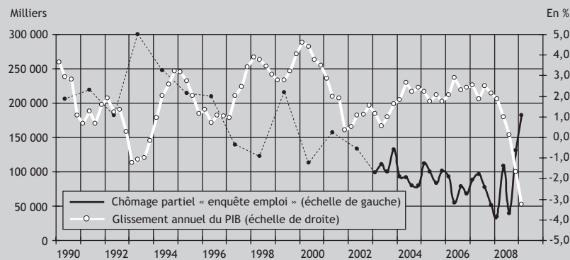
Nombre de personnes au chômage partiel selon l'« enquête Emploi » et glissement annuel du PIB
